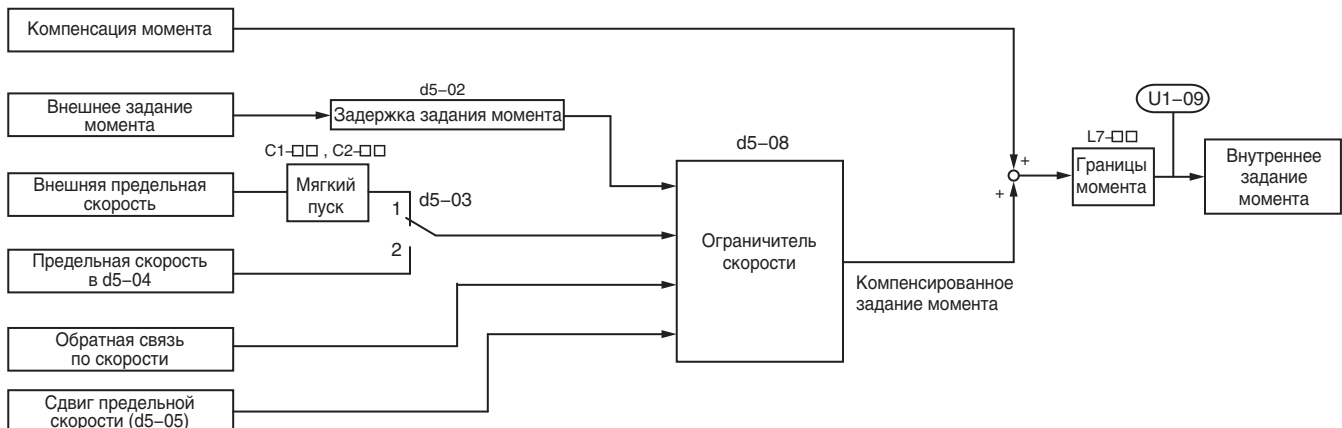
Рис. 5.50 Структурная схема функции регулирования вращающего момента
