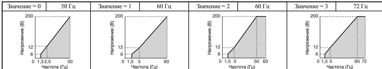
Табл. 5.30 Характеристики для постоянного крутящего момента, значения 0...3
