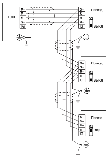
Рис. С.4 Интерфейс RS-422
