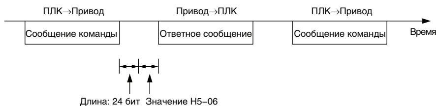
Рис. С.5 Настройка времени ожидания передачи привода
