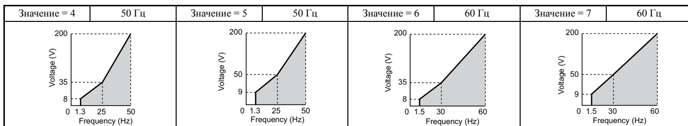
Табл. 5.24 Высокий пусковой момент, значения 8...В
