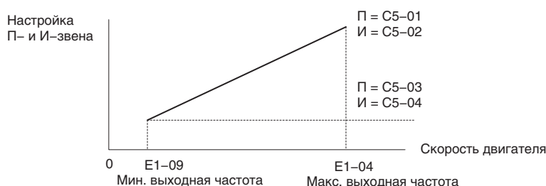
Рис. 5.37 Коэффициент передачи и время интегрирования ASR в режиме V/f с энкодером
