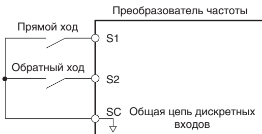
Рис. 5.63 Пример схемы подключения для 2-проводного управления
