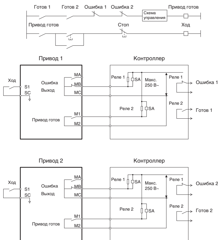
Рис. 3.32 Пример схемы блокировки
