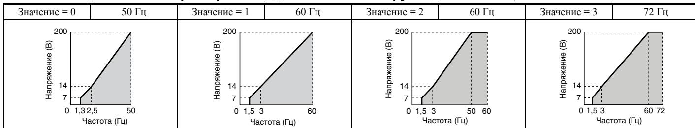
Табл. 5.27 Характеристики для пониженного крутящего момента, значения 4...7
