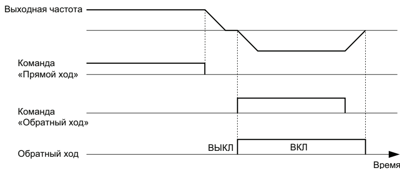
Рис. 5.75 Пример работы выхода сигнализации обратного направления
