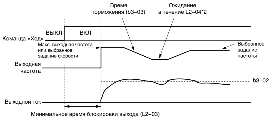
Рис. 5.18 Поиск скорости методом определения тока при пуске или по команде поиска скорости на дискретном входе
