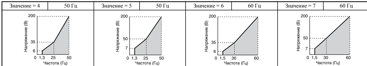
Табл. 5.28 Высокий пусковой момент, значения 8...B
