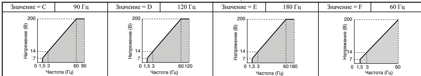
Табл. 5.29 Постоянное выходное напряжение, значения C...F
