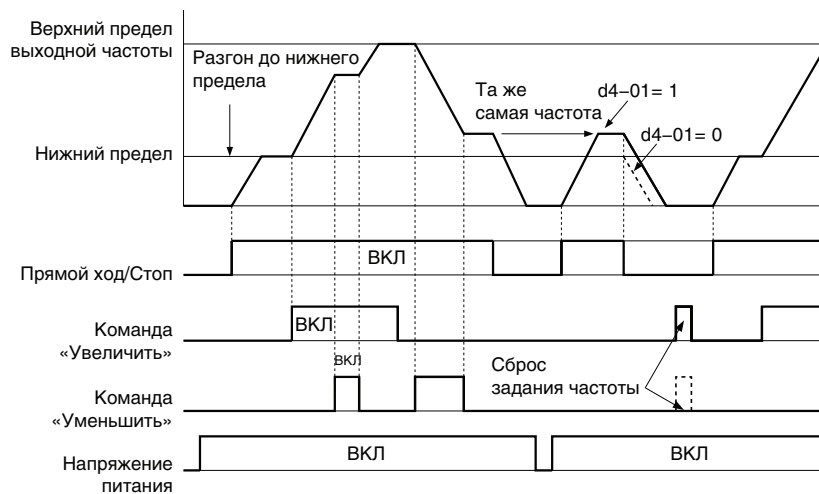
Рис. 5.58 Работа функции увеличения/уменьшения
