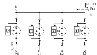
4-полюсные 5SD7 414-1
