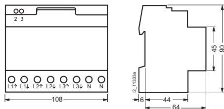
7KT1 3.0
