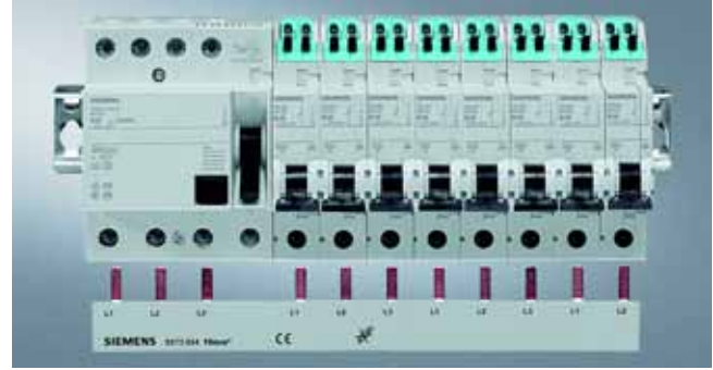
Подключение автоматических выключателей к 4-полюсному УЗО (N-зажим слева) распилываемой 3-полюсной сборной шиной из программы 5ST3 7..
