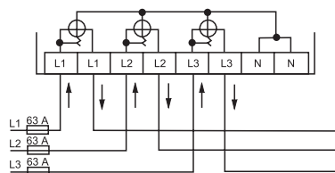
AC 400 В прямое подключение 63 А, 3-проводная схема
