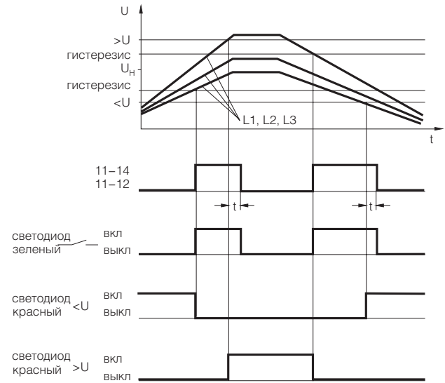
Временной график реле минимального/максимального напряжения 5TT3 408
