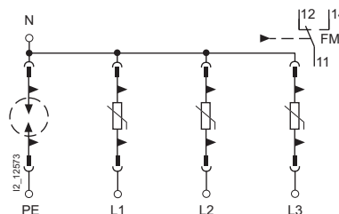
5SD7 424-0 без телесигнализации (FM)
