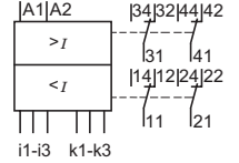
Пример принципиальной схемы 5TT6 114 с измерением через трансформатор
