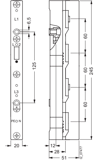
8US19 23-4AA00
