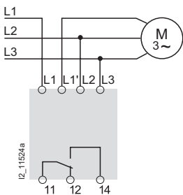
Подключение трехфазной нагрузки
