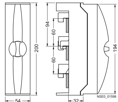
8US19 21-1BA00
