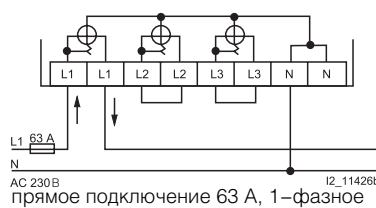
AC 230 В прямое подключение 63 А, 1-фазное
