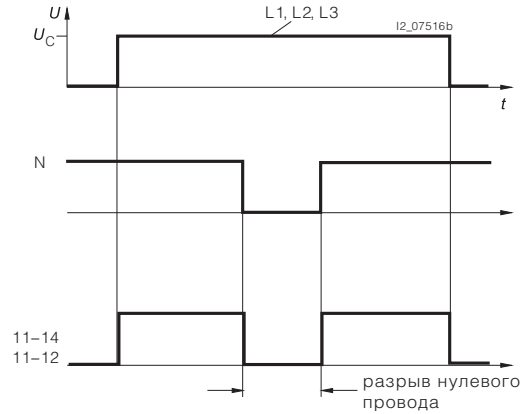
Временной график реле минимального/максимального напряжения 5TT3 408
