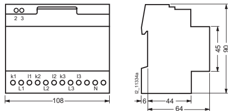
7KT1 3.2
