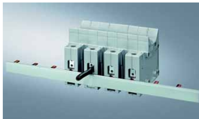
цоколи предохранителей 5SG1 301 сборная шина 5SG1 701 торцевые крышки 5ST3 703 5ST3 748
