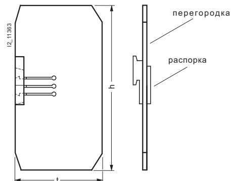
перегородка NH
