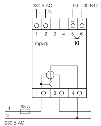
7КТ1 141
