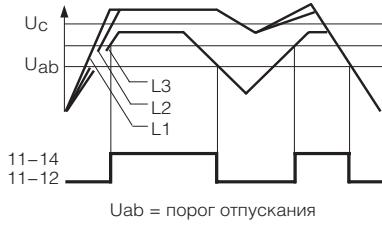
Временной график реле минимального напряжения 5TT3 400 - 5TT3 406
