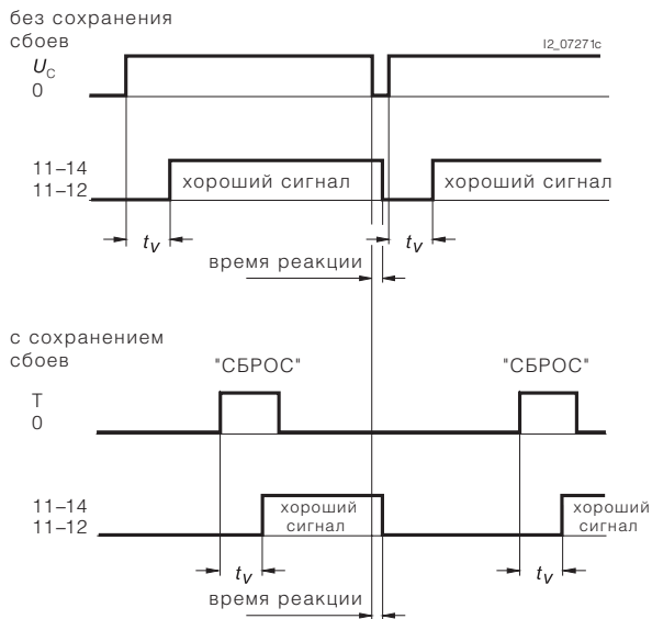
Временной график реле контроля кратковременного исчезновения напряжения 5TT3 407
