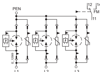
3-полюсные 5SD7 443-1
