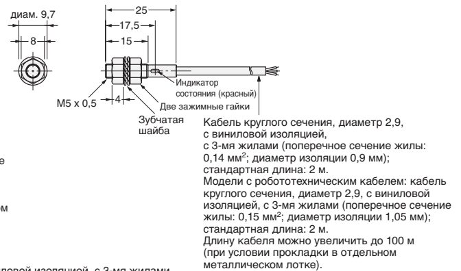
Рис. 3 : E2E-X1□□
