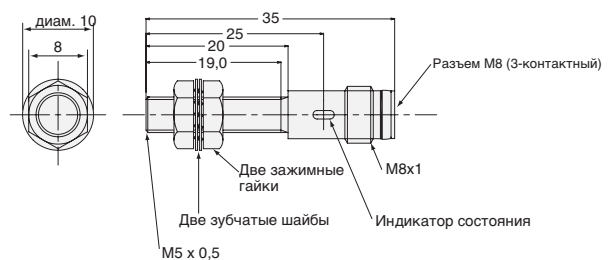
Рис. 36 : E2E-X1□□-M5
