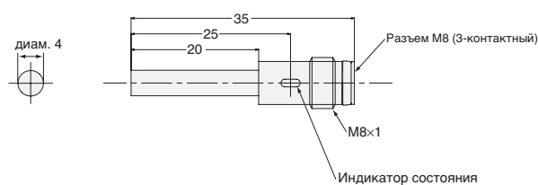
Рис. 35 : E2E-CR8□□-M5
