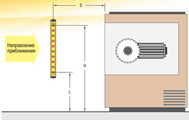
Датчик безопасности: ограждение опасного места Датчик безопасности: ограждение с трех сторон Датчики безопасности: ограждение по двум осям
