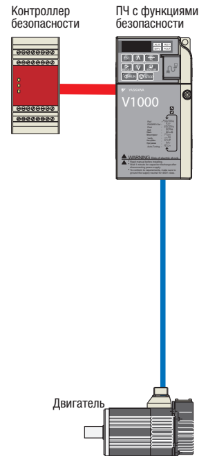
Схема безопасности с ПЧ с функцией безопасности
