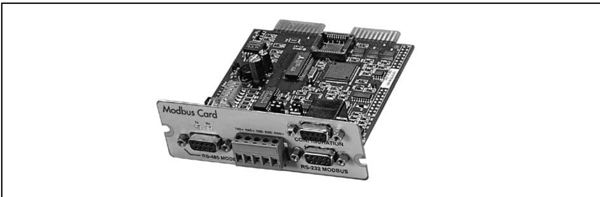
Рисунок 15 Модуль Modus/Jbus.
