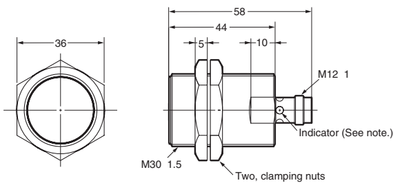
E2A-M30KS10-M1-□□/E2A-S30KS10-M1-□
