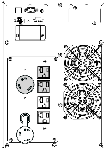
Рисунок 46. Модель PW9130L2000T-XL
