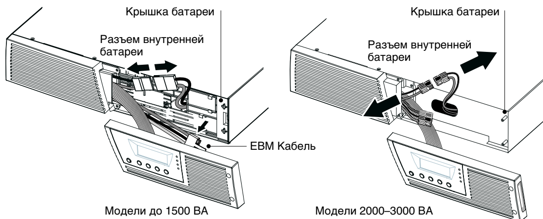
Рисунок 24. Отключение внутренних батарей ИБП (показано без EBM)
