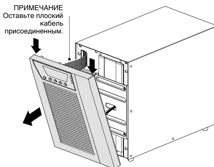
Рисунок 25. Снятие передней крышки ИБП
