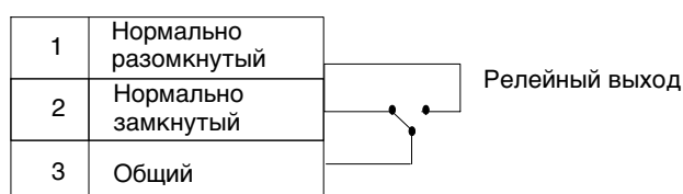
Рисунок 22. Стандартные подключения выходных портов
