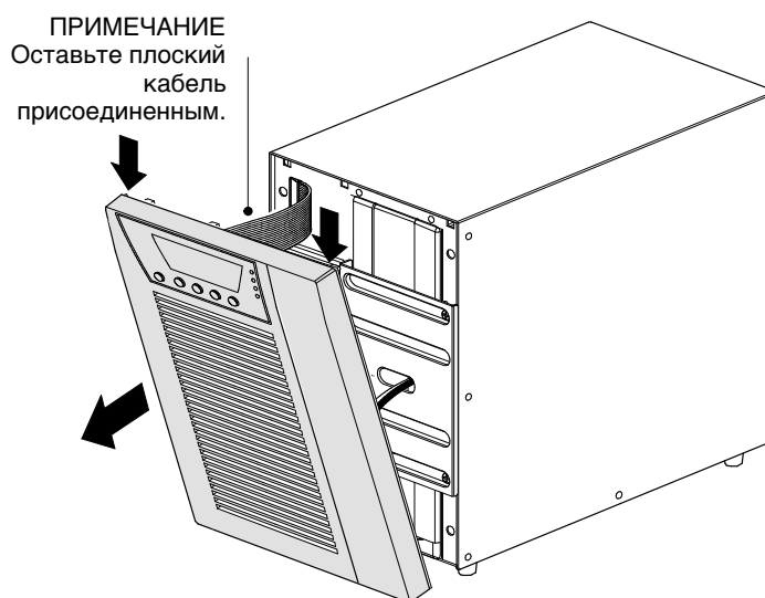
Рисунок 14. Снятие передней крышки ИБП
