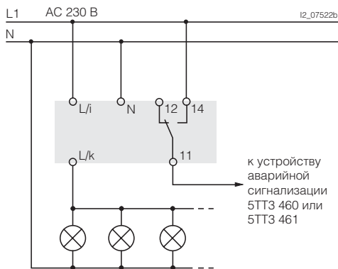
Пример принципиальной схемы реле минимального тока 5TT6 111
