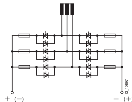
шестипульсовая мостовая схема B6 с предохранителями в ответвлениях (реверсивная схема)
