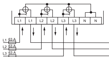
AC 400 V прямое подключение 63 А, 3-проводная схема
