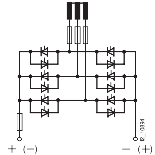
шестипульсовая мостовая схема B6 с фазными предохранителями и предохранителем постоянного тока (реверсивная схема)
