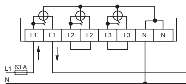
AC 230 V I2_11424 прямое подключение 63 А, 1-фазное
