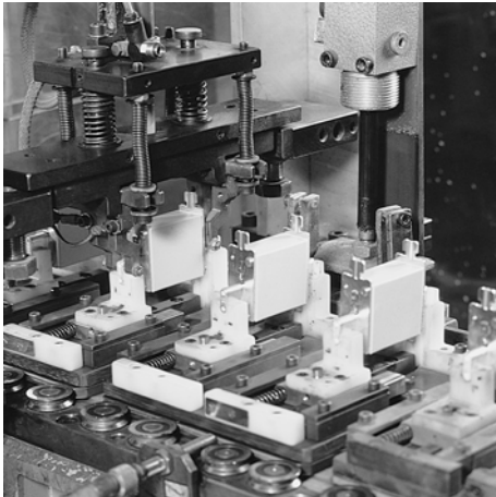
Линия производства плавких вставок предохранителей NH
