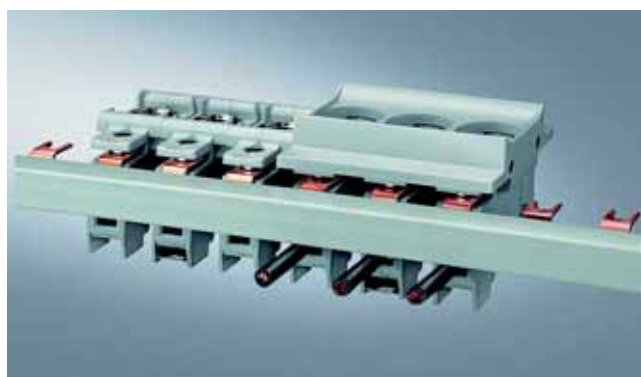
цоколи предохранителей 5SG5 330 сборная шина 5SG5 730 торцевые крышки 5SH5 320 5SH5 514
