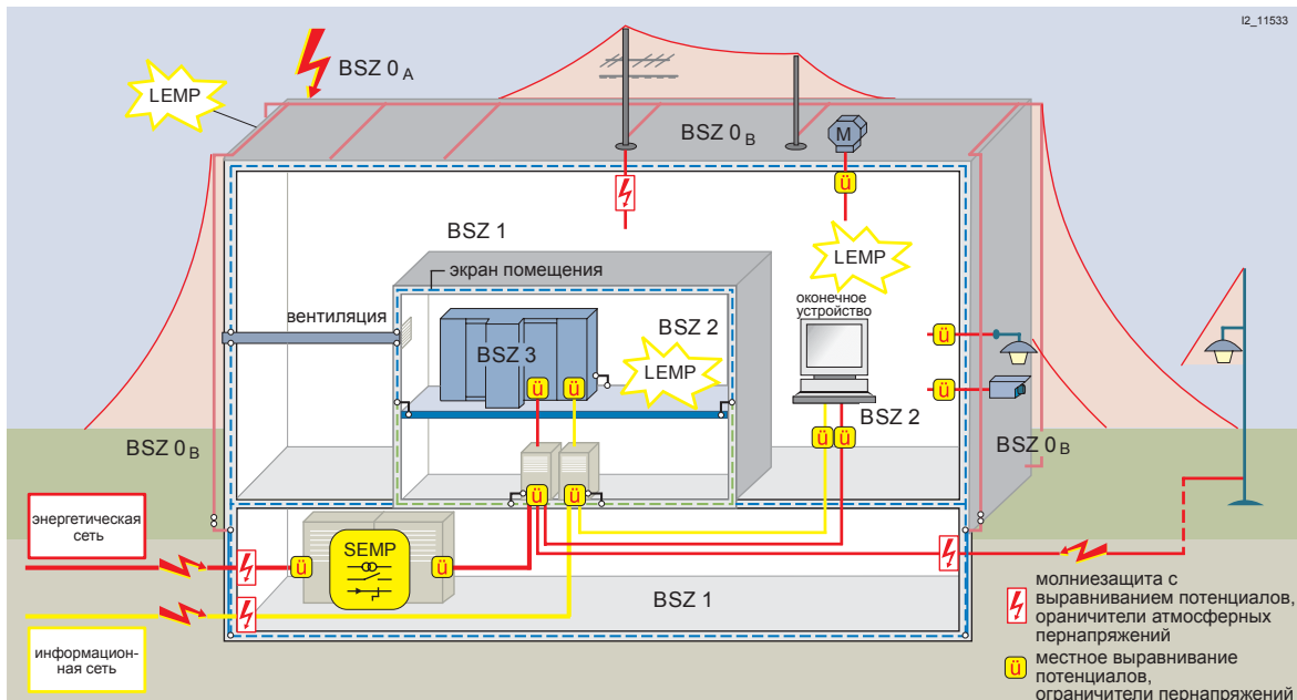
Концепция зон молниезащиты, соответствующая требованиям по электромагнитной совместимости
