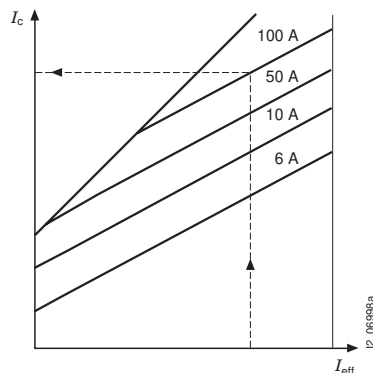
Диаграмма ограничения тока; Диаграмма тока отсечки предохранительных вставок NH типоразмер 00, класс использования gG, расчетные токи 6 А, 10 А, 50 А, 100 А
