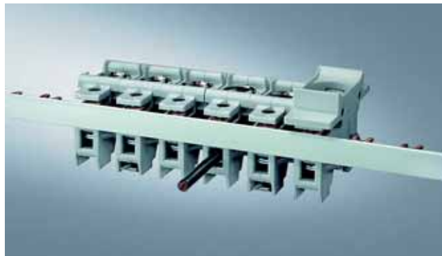
цоколи 5SG1 330 / 5SG1 331 5SG1 730 / 5SG1 731 сборная шина 5SH5 517 торцевые крышки 5ST3 748
