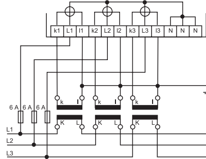
AC 400 В подключение через трансформаторы тока, 3-проводная схема
