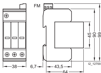
5SD7 423-0 без телесигнализации (FM)
