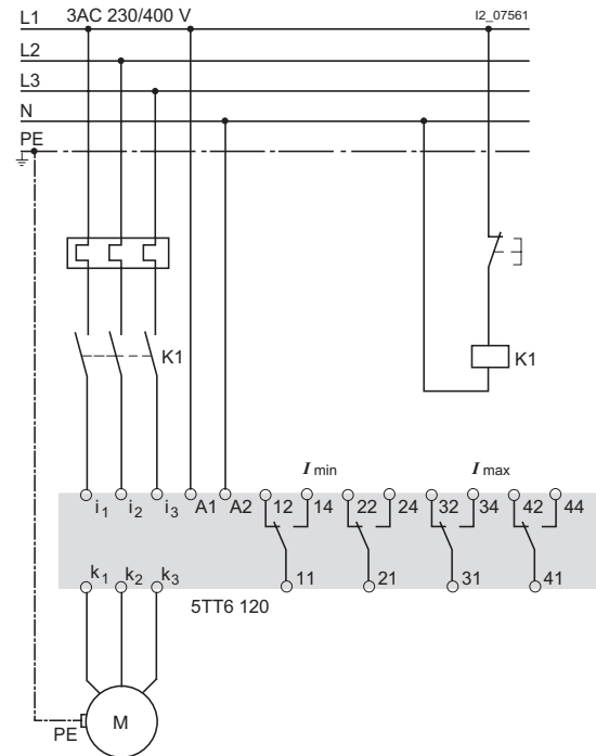
Пример принципиальной схемы 5TT6 120 с прямым измерением
