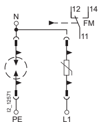
5SD7 422-0 без телесигнализации (FM)
