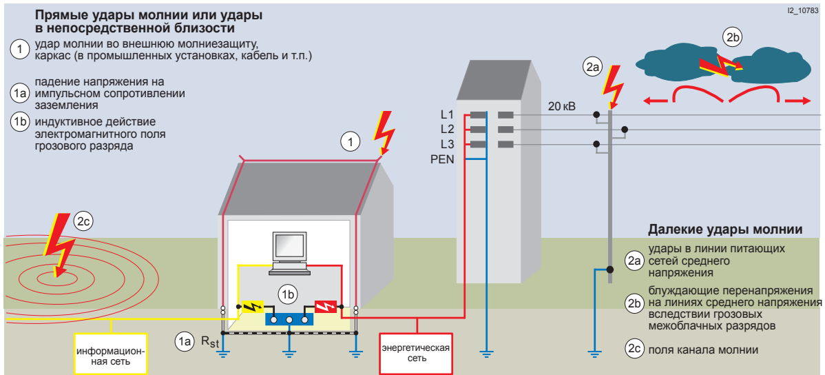
Причины перенапряжений при грозовых разрядах
