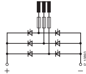
шестипульсовая мостовая схема B6 с фазными предохранителями
