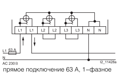
AC 400 В прямое подключение 63 А, 3-проводная схема
