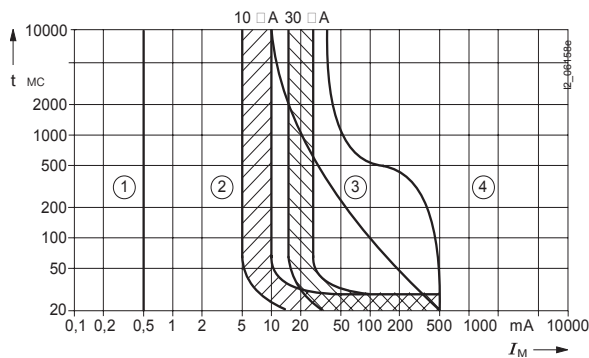
Диапазоны силы тока по МЭК 60 479
