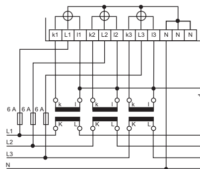
AC 230 / 400 V подключение через трансформаторы тока, 4-проводная схема
