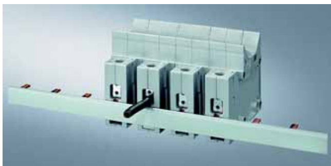
цоколи 5SG1 301, 5SG1 701 сборная шина 5ST3 703 торцевые крышки 5ST3 748
