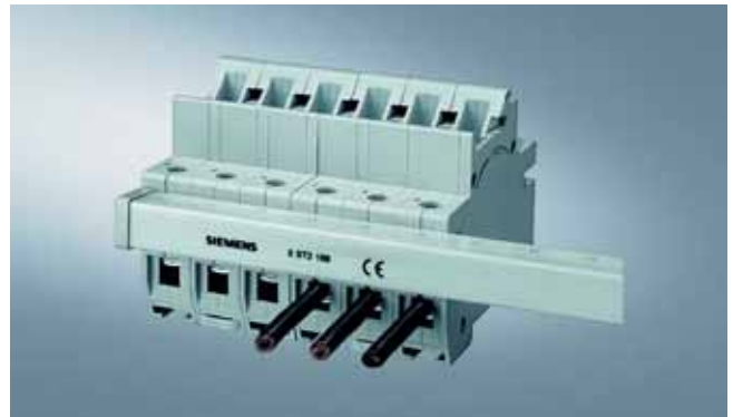
Предохранители-выключатели нагрузки 3-полюсные 5SG7 630 сборная шина 5ST2 188 или 5ST2 192 торцевые крышки 5ST2 177
