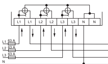
AC 230 / 400 V прямое подключение 63 А, 4-проводная схема
