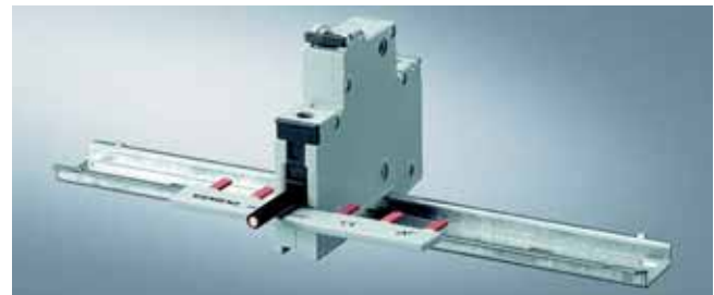
Большое доступное пространство для монтажа Видимое, однозначное и контролируемое подключение проводов
