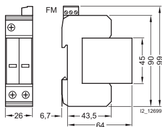
5SD7 422-0 без телесигнализации (FM)
