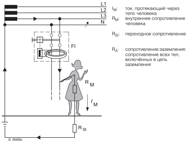
Принципиальная схема: Дополнительная защита при прямом прикосновении к токоведущим частям
