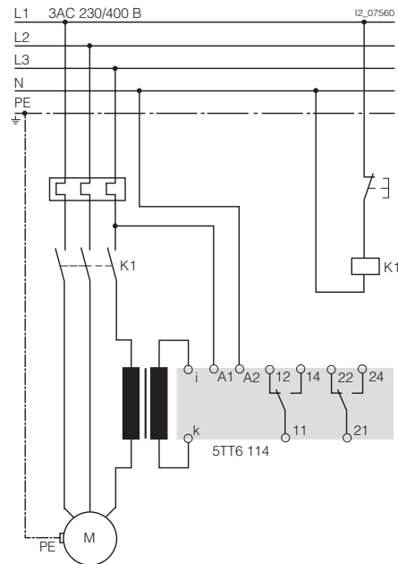
Пример принципиальной схемы 5TT6 114 с измерением через трансформатор
