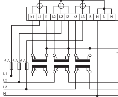
AC 230 / 400 В подключение через трансформаторы тока, 4-проводная схема
