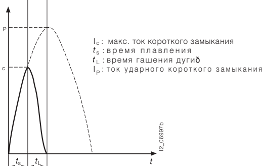
Осциллограмма отключения тока короткого замыкания плавкой вставкой предохранителя
