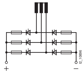
шестипульсовая мостовая схема B6 с предохранителями в ветвях
