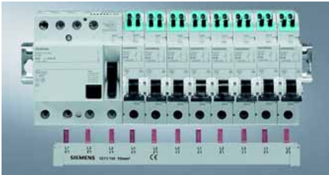
Подключение автоматических выключателей к 4-полюсному УЗО (N-зажим справа) 3-полюсной сборной шиной заводского изготовления из программы 5ST3 6..
