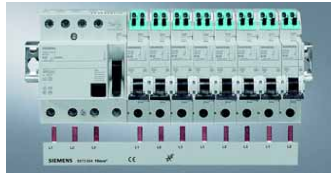
Подключение автоматических выключателей к 4-полюсному УЗО (N-зажим слева) распиливаемой 3-полюсной сборной шиной из программы 5ST3 7..
