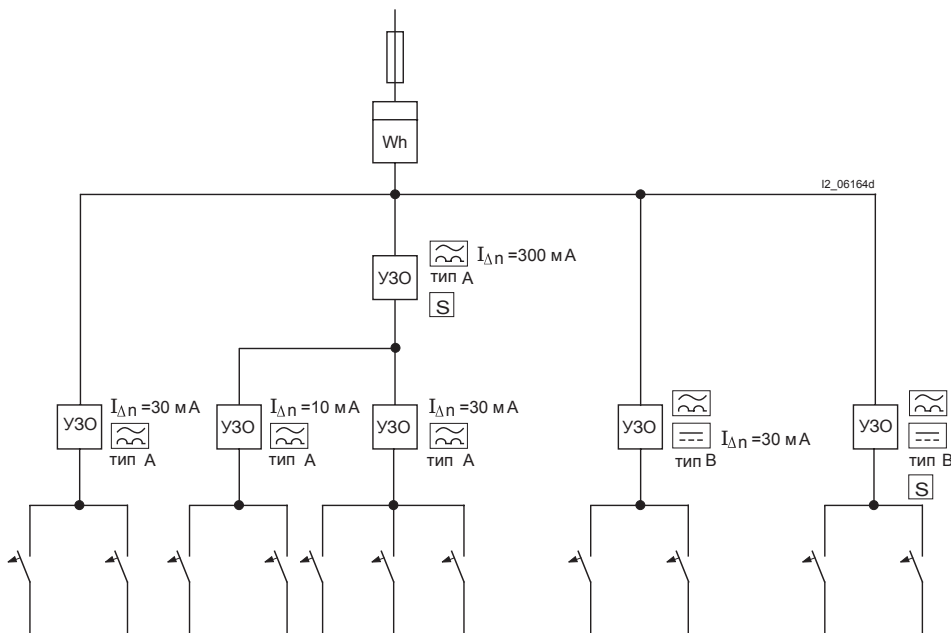
Пример проектирования с устройствами защитного отключения, тип А и тип В
