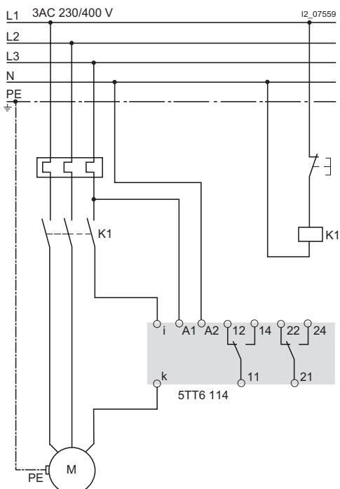
Пример принципиальной схемы 5TT6 114 с прямым измерением
