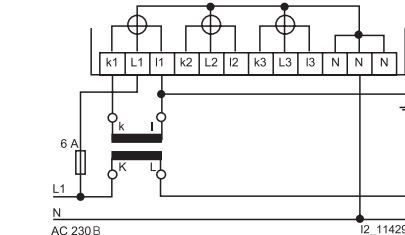
AC 230 В подключение через трансформаторы тока, 1-фазное
