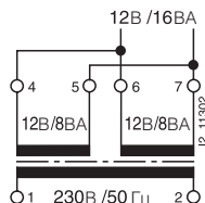
4AC2 961-6 параллельное соединение
