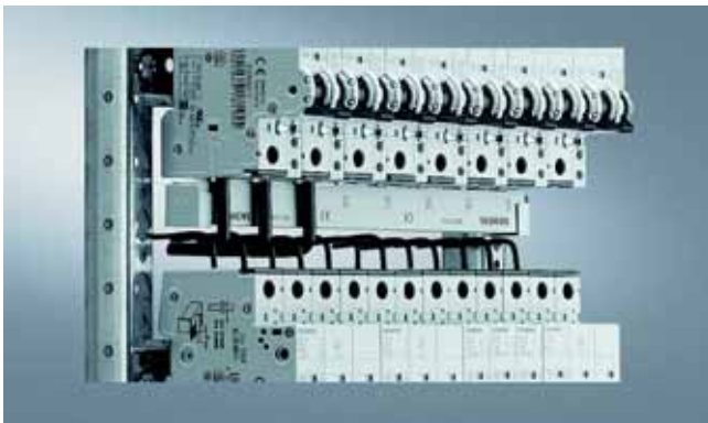
Оптимальное пространство для монтажа также и при малых расстояниях между монтажными рейками
