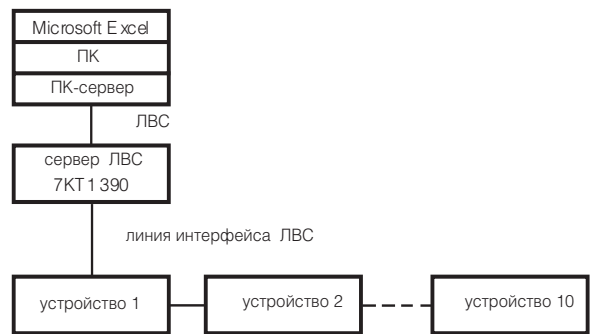
Блок-схема установки
