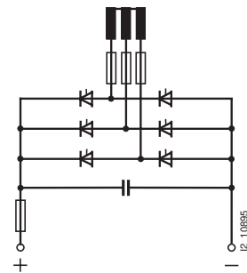
шестипульсовая мостовая схема B6 с фазными предохранителями и предохранителем постоянного тока (схема для преобразователя частоты переменного тока)
