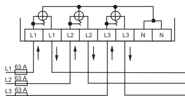
AC 400 В прямое подключение 63 А, 3-проводная схема
