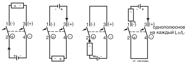
До напряжения аккумуляторной батареи макс. DC 220 В
