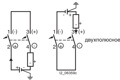
До напряжения аккумуляторной батареи макс. DC 440 В
