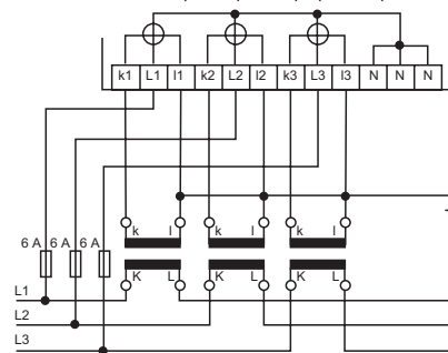
AC 400 V подключение через трансформаторы тока, 3-проводная схема
