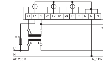
AC 230 В подключение через трансформаторы тока, 1-фазное
