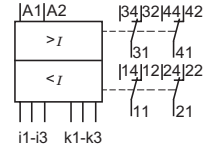
Пример принципиальной схемы 5TT6 114 с измерением через трансформатор
