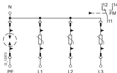
5SD7 424-0 без телесигнализации (FM)
