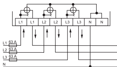
AC 230 / 400 В прямое подключение 63 А, 4-проводная схема
