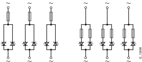
трехфазная схема переключения W3 с предохранителями в фазах с предохранителями в ветвях
