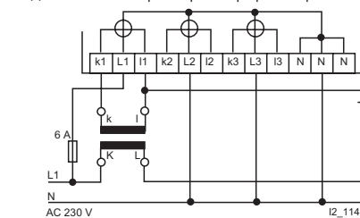
AC 230 V I2_11425 подключение через трансформаторы тока, 1-фазное
