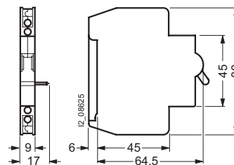
Блок-контакт 5ST3 018-0KV/ сигнализатор срабатывания 5ST3 028-0KV
