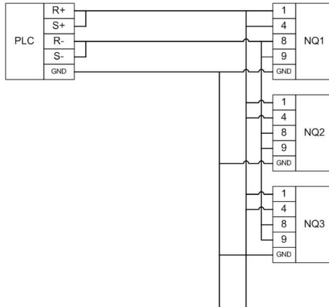
Рис. 3.11: Сеть RS-485
