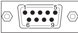
Разводка контактов вилки DB9 (ПЛК)
