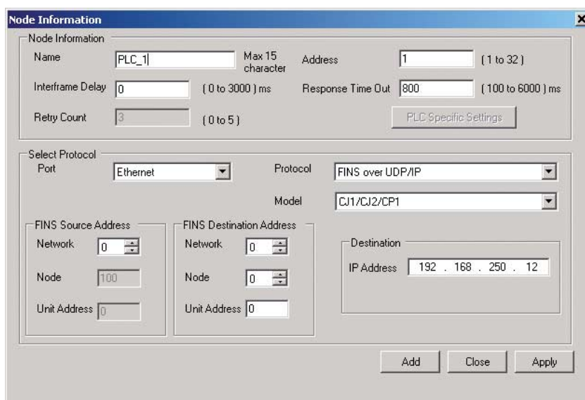
Рис. 4.33: Информация об узле
