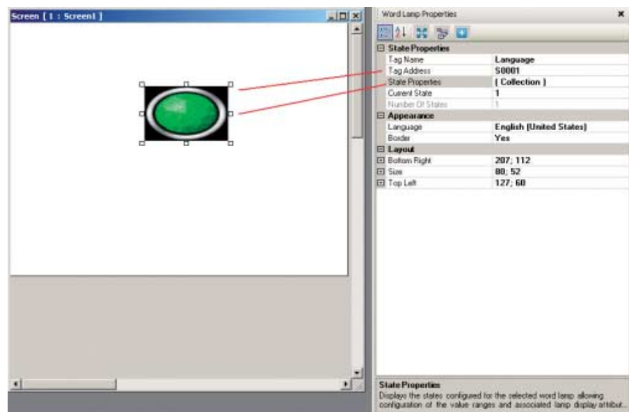
Рис. 4.22: Лампы
