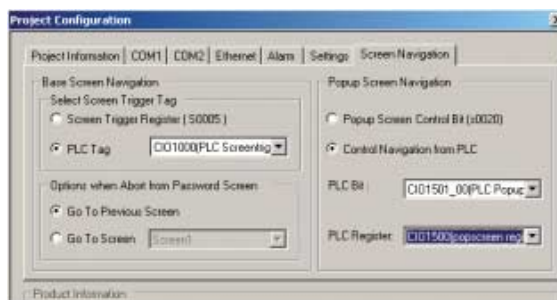
Рис. 4.14: Вкладка «Переключение экранов» (Screen Navigation)
