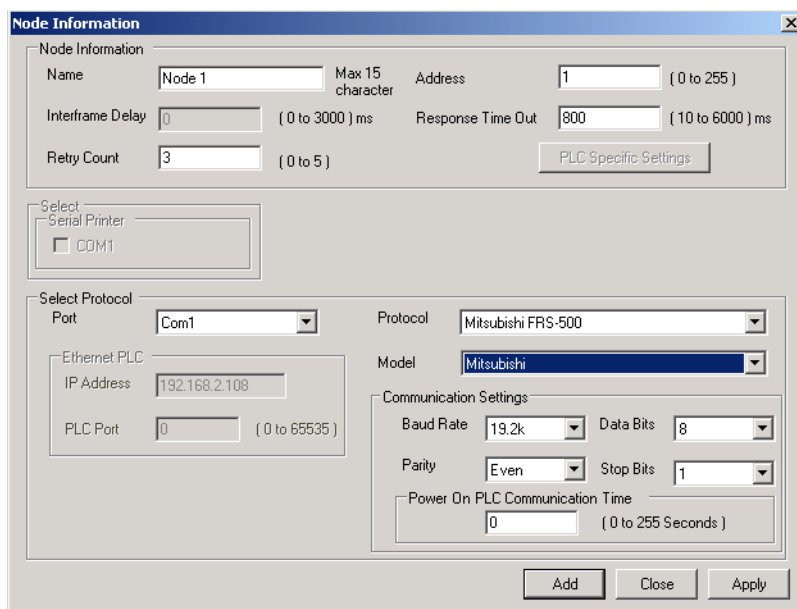
Рис. А.27: Информация об узле
