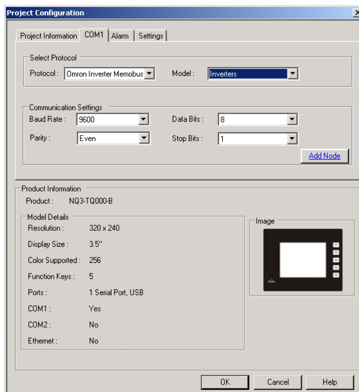
Рис. 4.46: Конфигурация проекта
