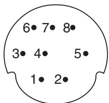
Разводка контактов 8-конт. разъема MINI DIN (ПЛК)
