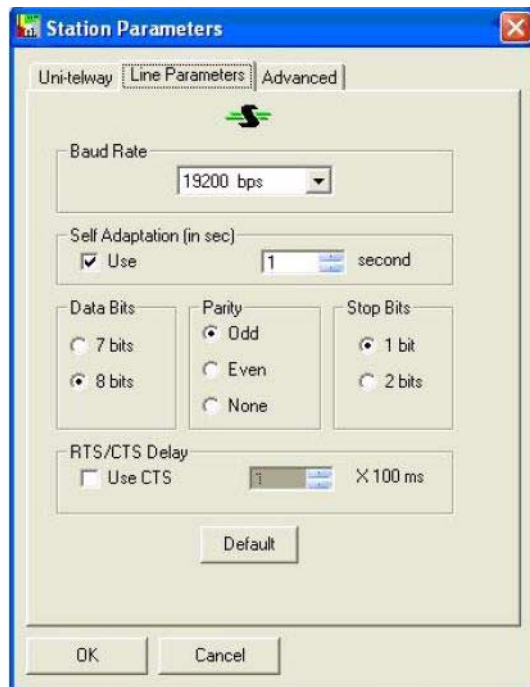
Рис. А.39: Параметры станции
