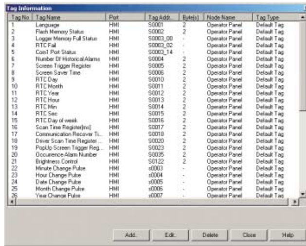
Рис. 4.4: Информация о тегах
