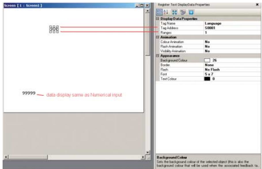
Рис. 4.18: Объекты отображения данных
