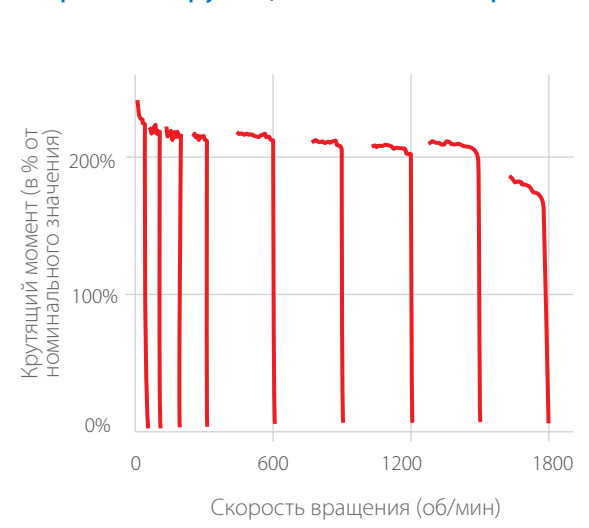
(Пример зависимости характеристик скорости и крутящего момента: серия RX)
