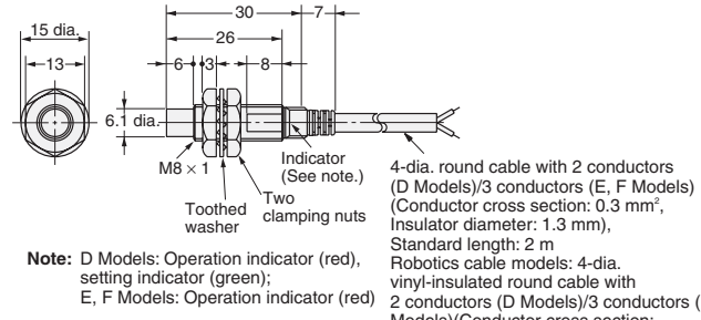
Fig. 5 : E2E-X4MD□ E2E-X2ME□/F□
