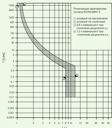
Кривая отключения BZM2 160A, 3 x полюсное исполнение
