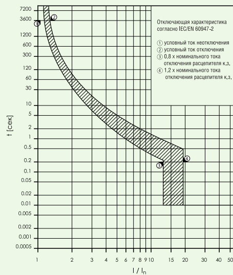
Кривая отключения BZM1 32A, 3 x полюсное исполнение
