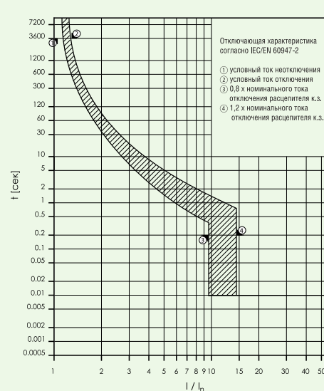
Кривая отключения BZM1 50A, 3 x полюсное исполнение
