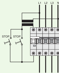
Пример соединения 24 В
