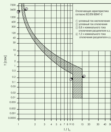
Кривая отключения BZM1 50A, 3 x полюсное исполнение
