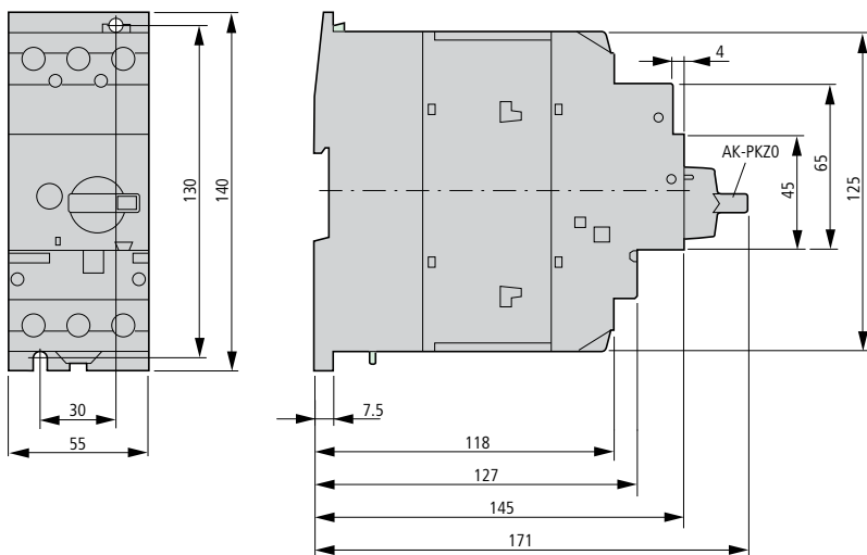
Трехфазные соединители B3.0/4-PKZ4
