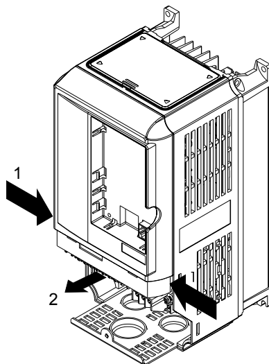
Рис. 1.17 Снятие передней крышки (на примере модели CIMR-E7Z45P5)
