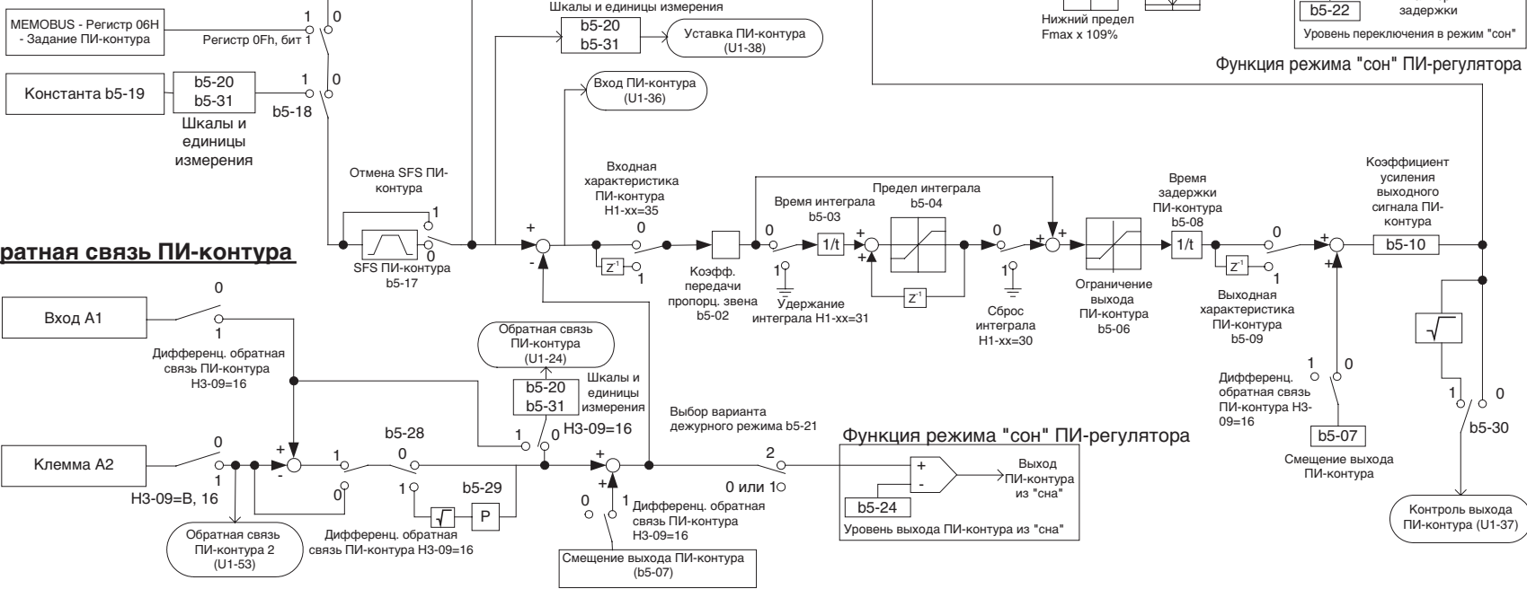
Рис. 6.57 Схема блока ПИ-регулятора
