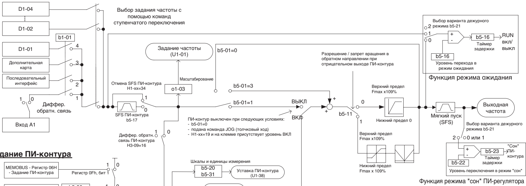
Рис. 6.57 Схема блока ПИ-регулятора
