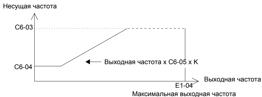
Рис. 6.4 Коэффициент масштабирования несущей частоты
