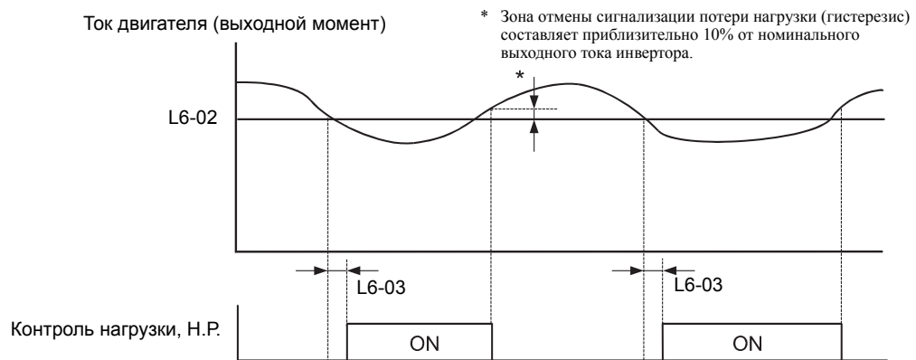
Рис. 6.28 Пример работы функции обнаружения потери нагрузки
