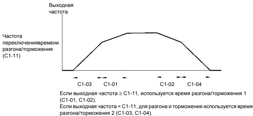
Рис. 6.18 Переключение времени разгона/торможения по частоте
