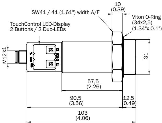
UP56-211/ 212/ 213
