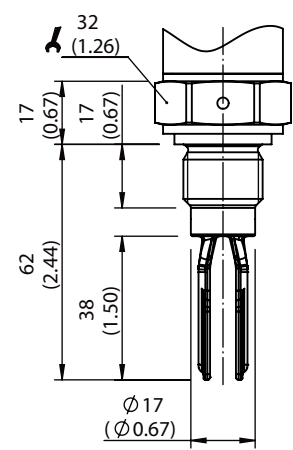
G ½ A, ½" NPT
