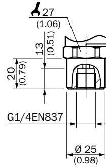
G 1/4 female EN 837
