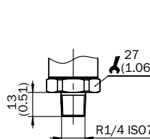
R 1/4 ISO 7
