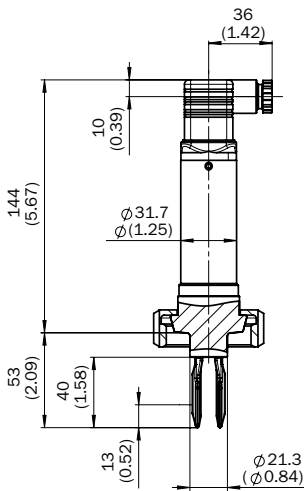
DIN 11851 DN 25, DN 40, DN 50; DIN 43650 incl. plug angled/IP 65
