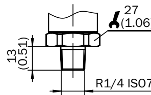
R 1/4 ISO 7
