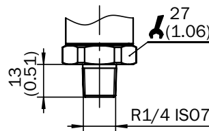
R 1/4 ISO 7
