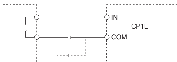
Релейный выход
