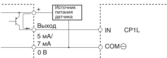
Токовый PNP-выход
