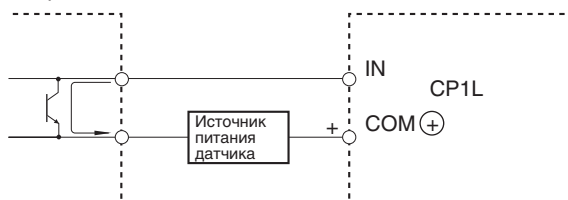
2-пров. выход пост. тока
