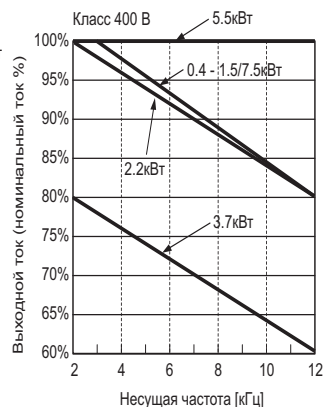
(3) Установка "стенка к стенке" (температура окружающей среды: 40°C)
