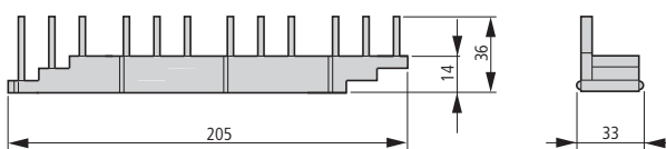
Трёхфазные соединители B3.0/4-PKZ4
