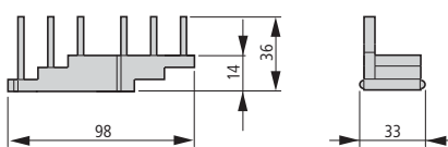
B3.0/2-PKZ4
