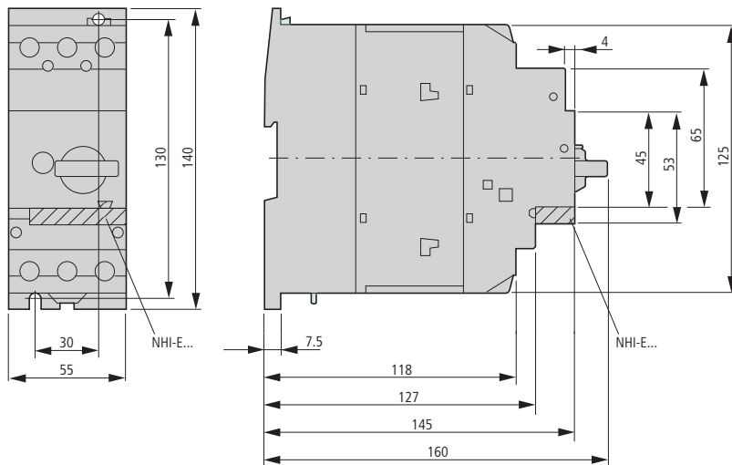
Автоматические выключатели защиты двигателей PKZM4-...
