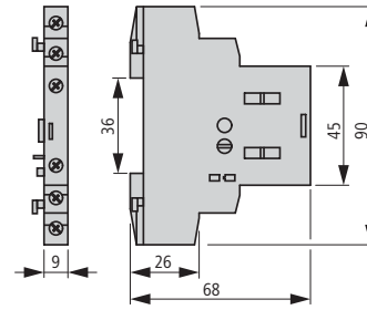
Стандартные вспомогательные контакты NHI...-PKZ... NHI...-PKZO
