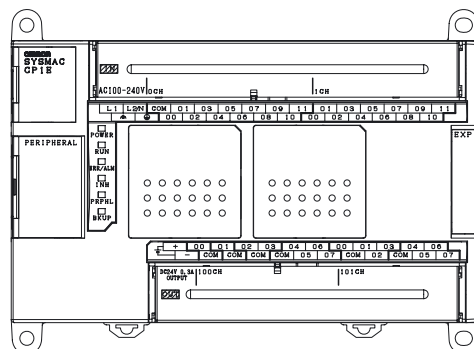
Модуль ЦПУ типа E CP1E-E40DR-A
