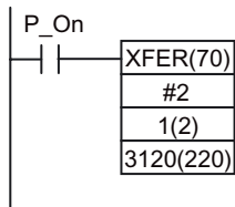
Котел С CP1L (ведом. устр-во 1)
