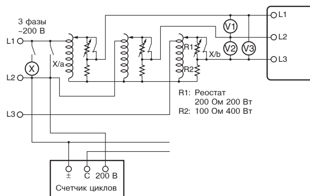
Схема подключения
