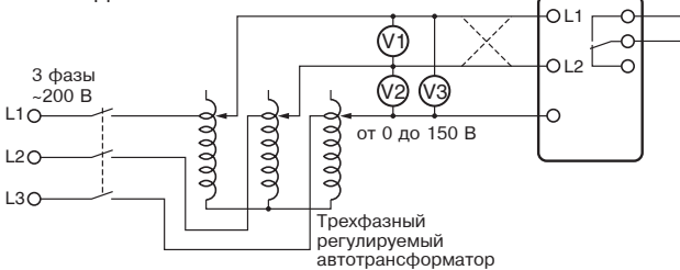
Схема подключения 1
