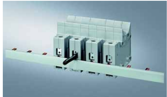
цоколи предохранителей 5SG1 301 сборная шина 5SG1 701 торцевые крышки 5ST3 703 5ST3 748
