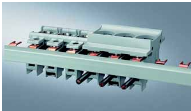
цоколи предохранителей 5SG5 330 5SG5 730 сборная шина 5SH5 320 торцевые крышки 5SH5 514
