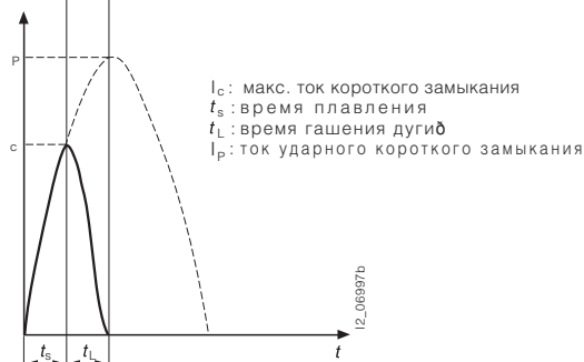
Осциллограмма отключения тока короткого замыкания плавкой вставкой предохранителя
