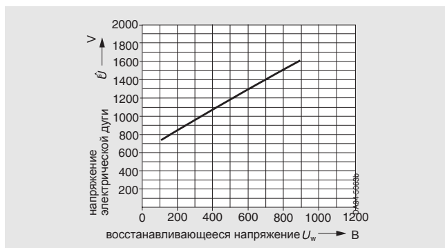
Пример: предохранительная вставка SITOR 3NE4 333-0B
