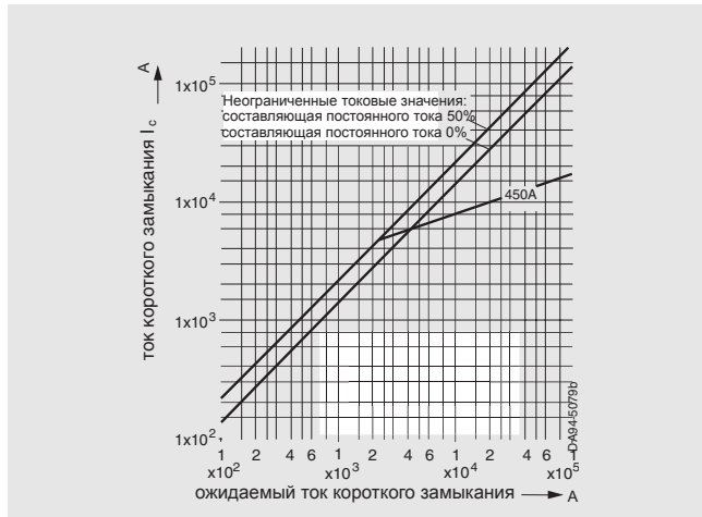
Пример: предохранительная вставка SITOR 3NE4 333-0B
