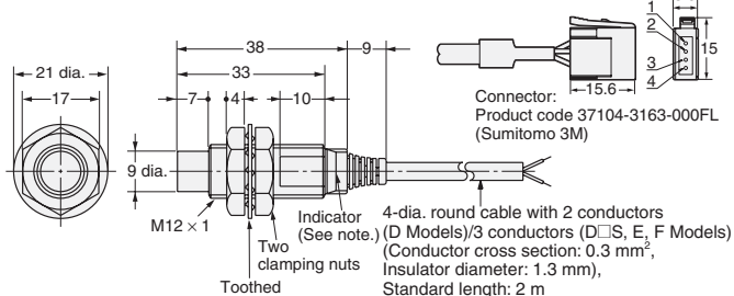
Fig. 9 : E2E-X8MD□ E2E-X5ME□/F□
