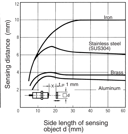
E2E-X10ME□/F□ E2E-X10MY□
