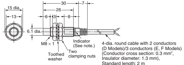
Fig. 5 : E2E-X4MD□ E2E-X2ME□/F□
