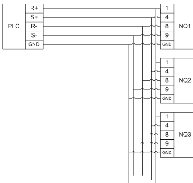
Рис. 3.10: Сеть RS-422
