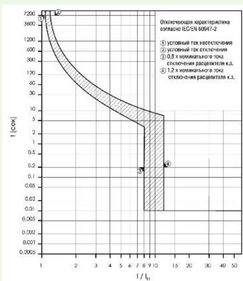
Кривая отключения BZM2 200A, 3 x полюсное исполнение
