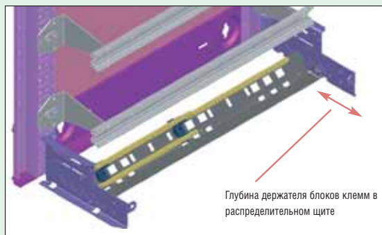
Деталь
