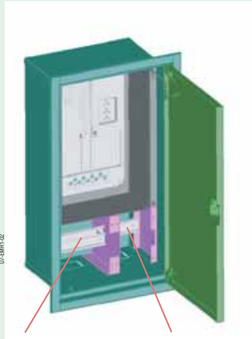
Приборная рейка для неизмеряемой части (8 модулей) Приборная рейка для измеряемой части
