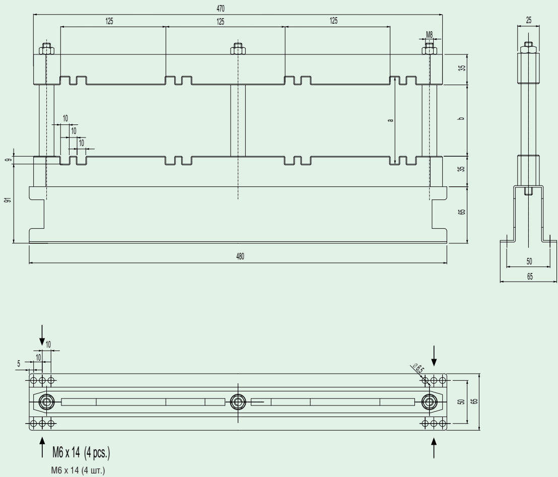
Размеры [мм]
