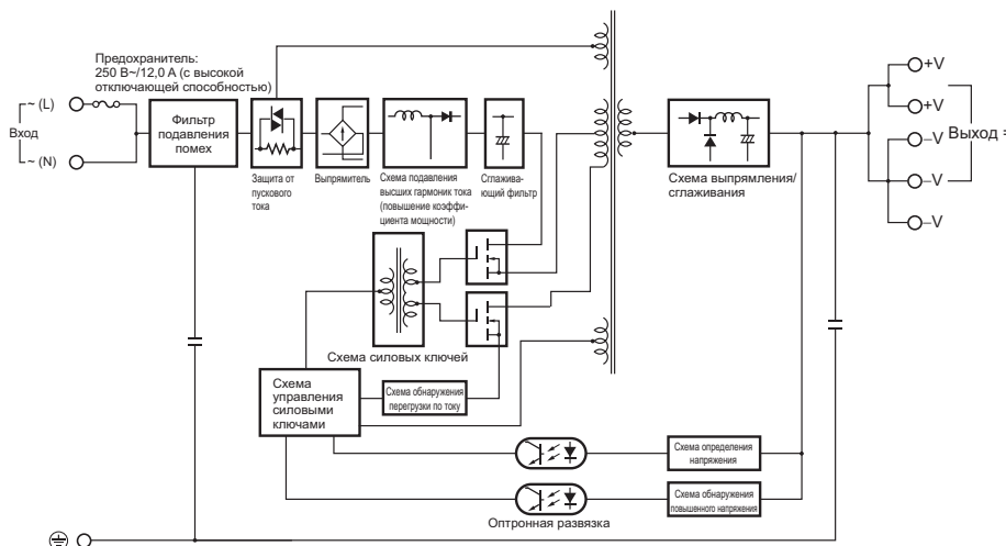
S8VK-C48024 (480 Вт)
