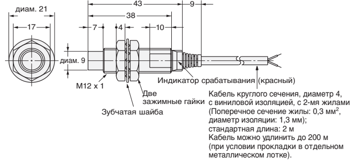
Рис. 6: E2E-X10MY□
