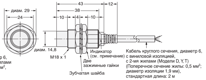
Рис. 6: E2E-X10MY□
